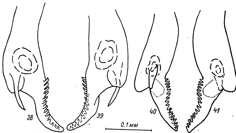
Рис. 38—41. Вершина эдеагуса..
