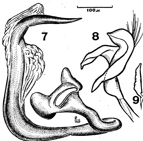
Platyscytus peruvianus n. sp. — Fig. 7: Pênis; fig. 8: parâmero esquerdo; fig. 9: parâmero direito.
